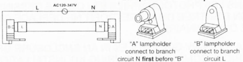
Figure 1. - Double-Ended connection (Figure 1. - Connexion à double extrémité)
