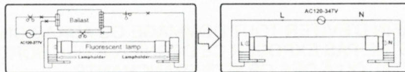
Figure 2. - Retrofit with One Lamp (Figure 2. - Installation avec une lampe)
