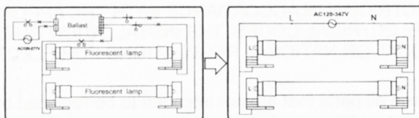
Figure 3. - Retrofit with Two Lamps (Figure 3. - Installation avec deux lampes)
